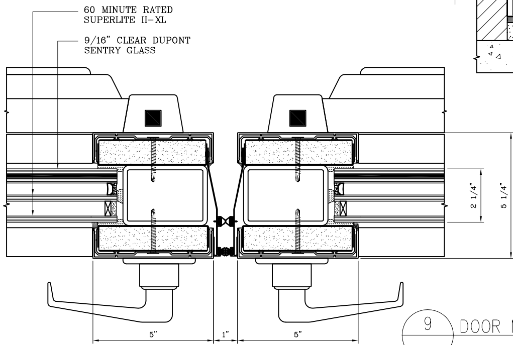
7 DOOR BOTTOM RAIL DETAIL
