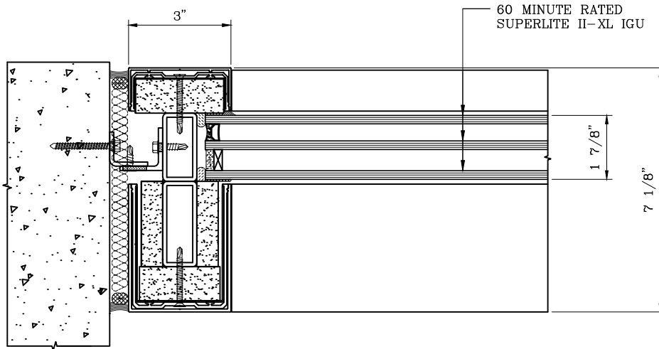
① JAMB DETAIL
