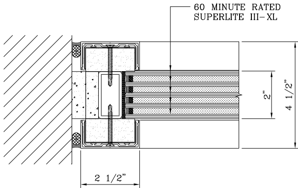
1 JAMB DETAIL
