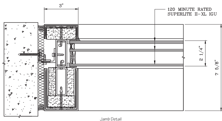
Jamb Detail
