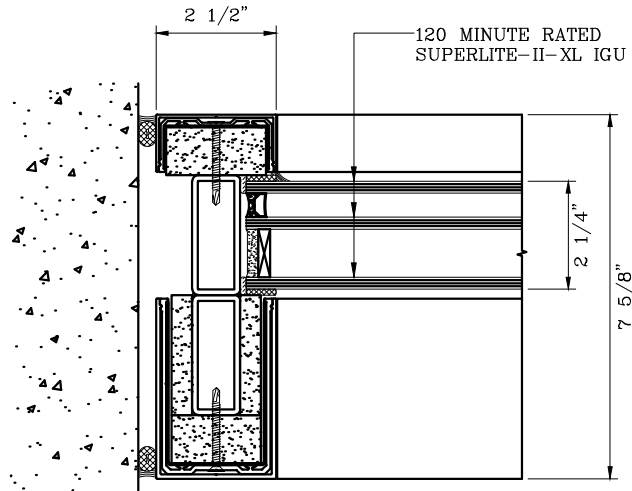
1 JAMB DETAIL
