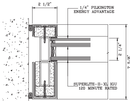
JAMB DETAIL
