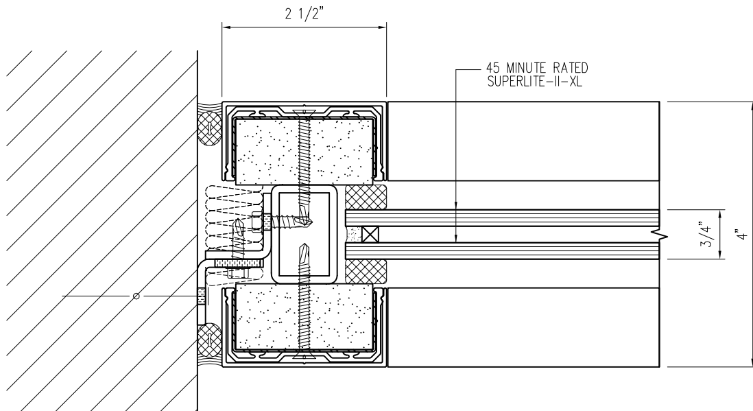
37a JAMB DETAIL 60 GPX-0-45R-IIXL
