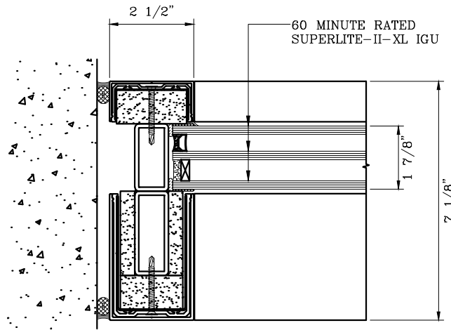
1 JAMB DETAIL
