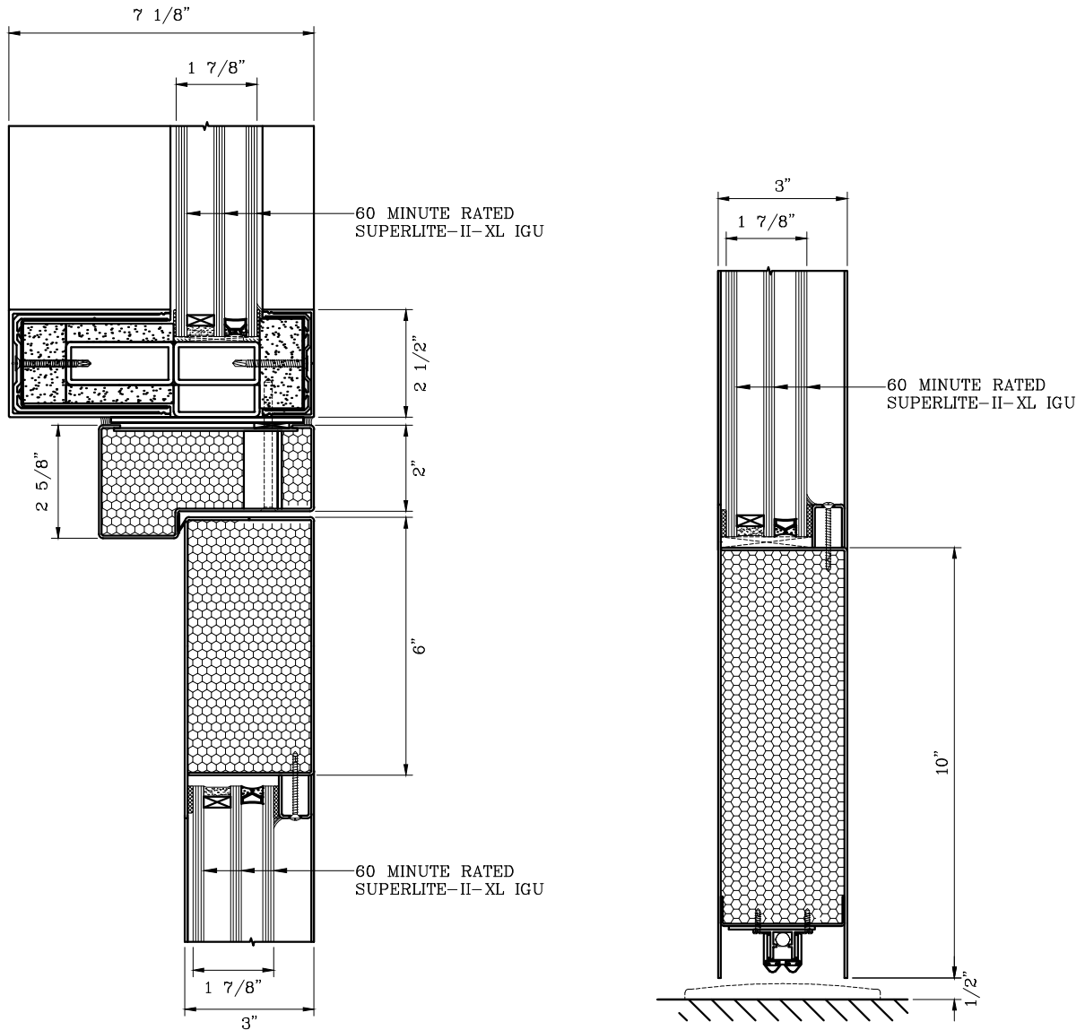
6 DOOR TOP RAIL DETAIL
