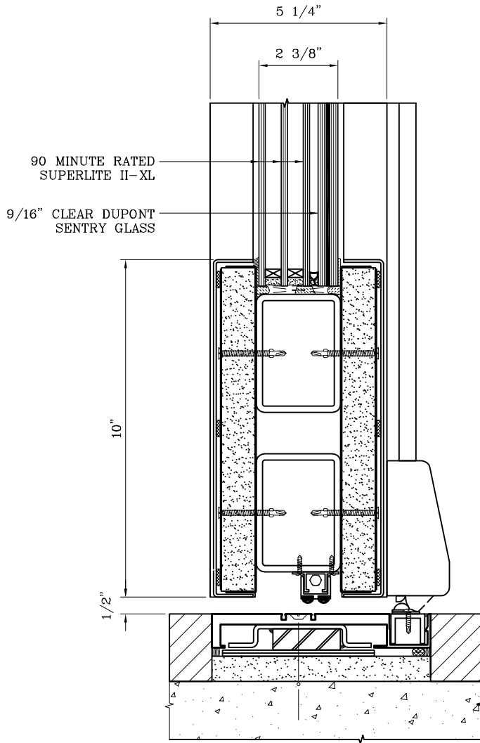
7 DOOR BOTTOM RAIL DETAIL
