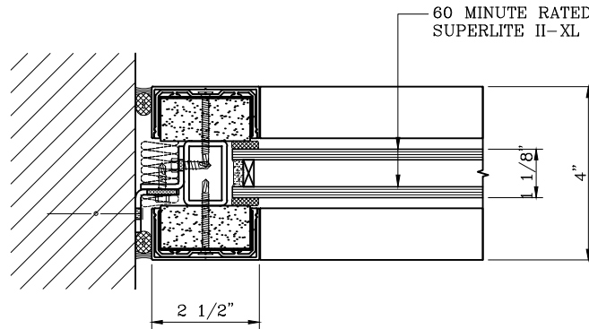
1 JAMB DETAIL -
