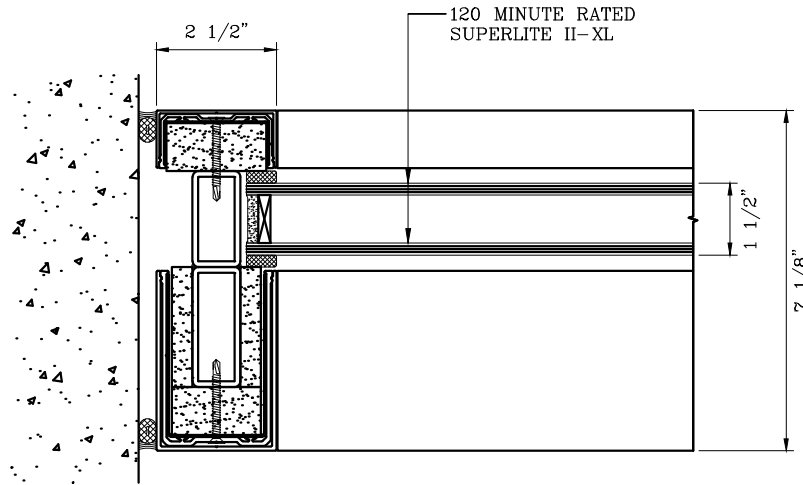
1 JAMB DETAIL
