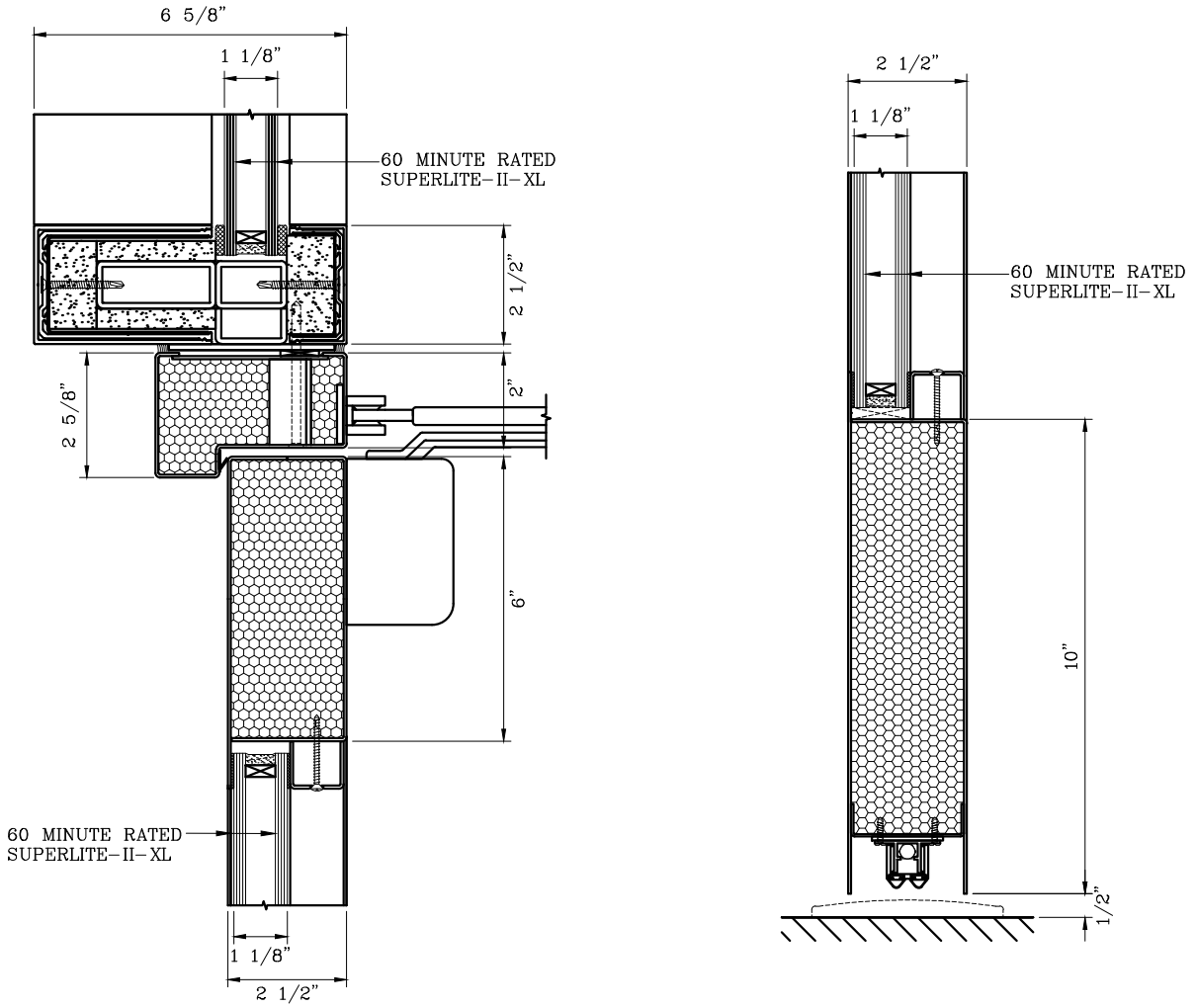
6 DOOR TOP RAIL DETAIL
