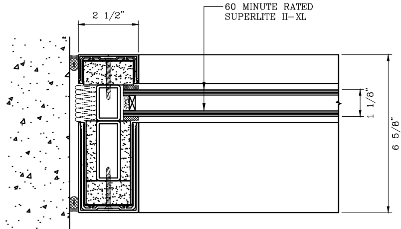
1 JAMB DETAIL
