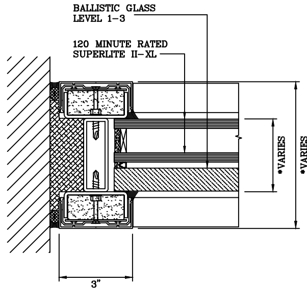
1 JAMB DETAIL
