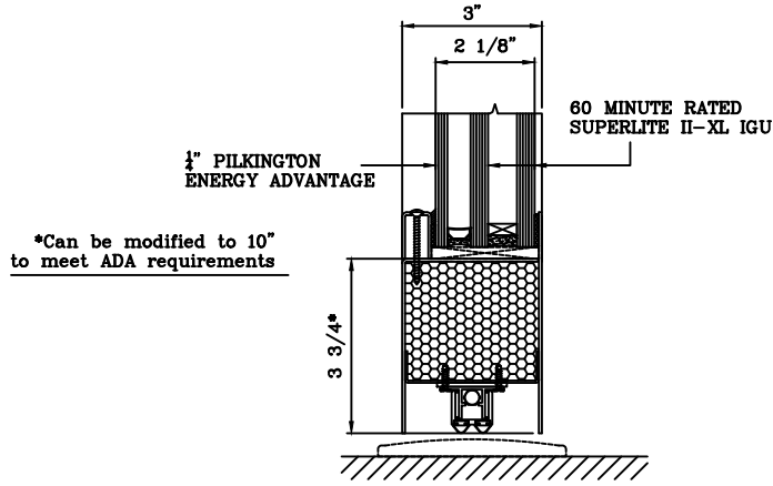
7 DOOR BOTTOM RAIL DETAIL
