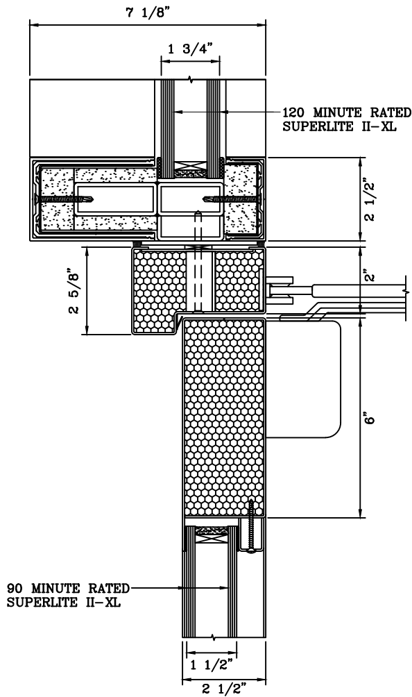
6 — DOOR TOP RAIL DETAIL
