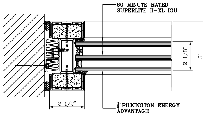
1 JAMB DETAIL
