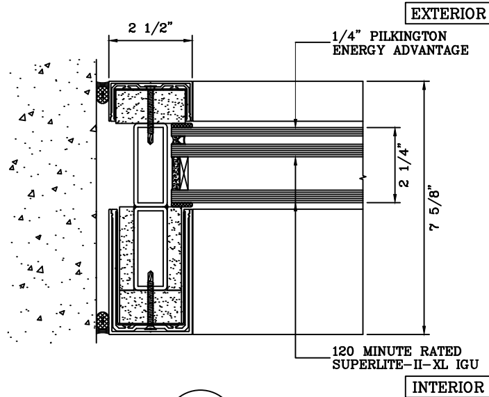
1 JAMB DETAIL
