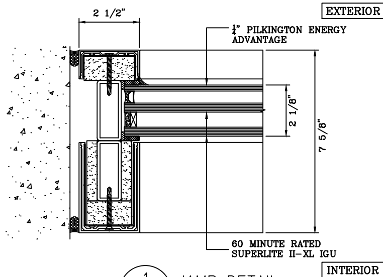
1 JAMB DETAIL
