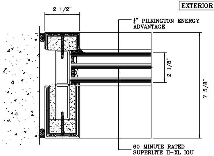
1 JAMB DETAIL EXTERIOR
