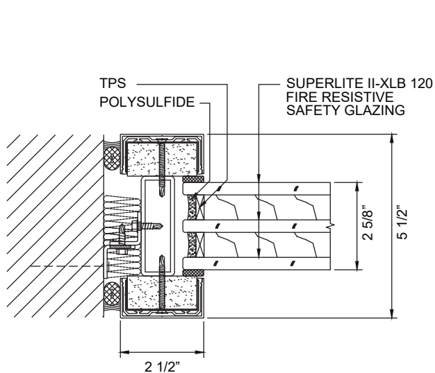
JAMB DETAIL
