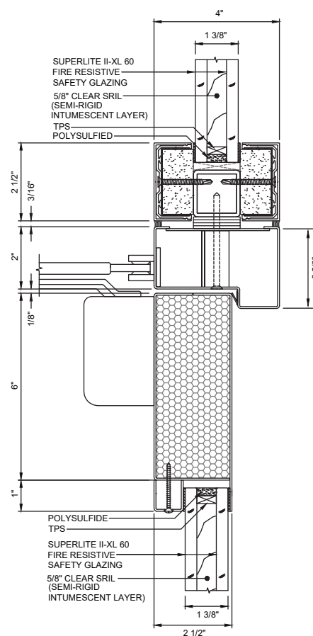
DOOR TOP RAIL DETAIL
